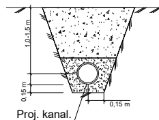
PE CAURULES MONTĀŽAS SHĒMA
