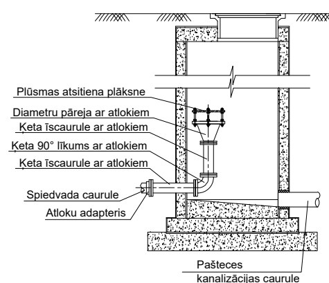
PIEVIENOŠANĀS PIE ESOŠAS SPIEDIENA DZĒŠANAS AKAS, B/M
